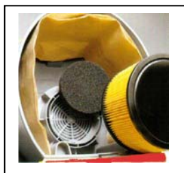
3-fach Filtersystem Staubbehälter
